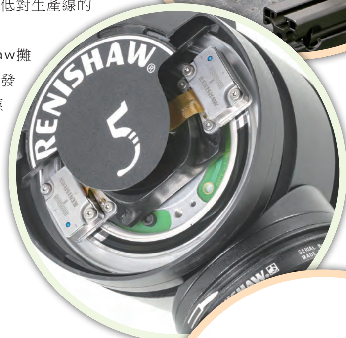
搭載 ATOM 光學尺的 REVO 5 軸三次元測頭。 Renishaw
