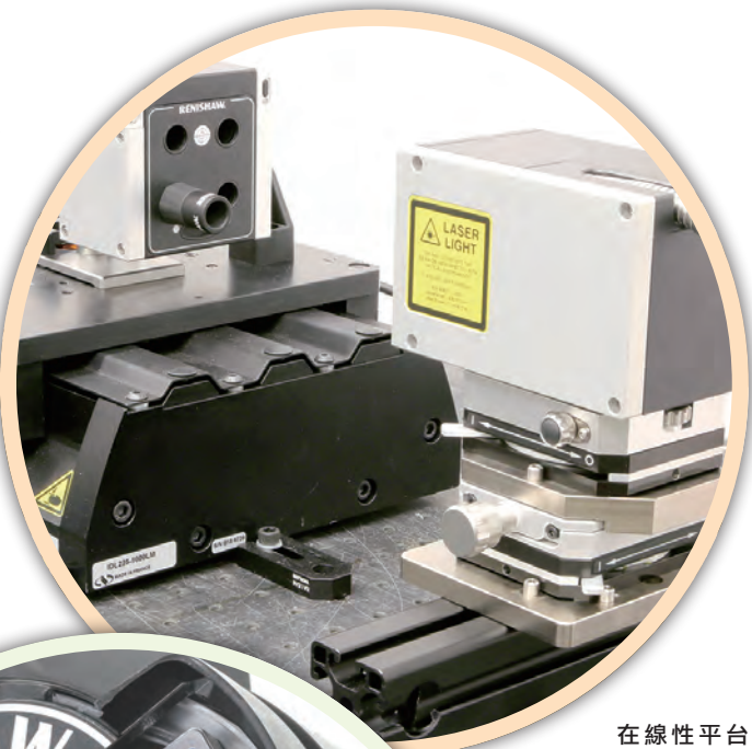
在線性平台上的 XM-60 多光束校正儀。 Renishaw
